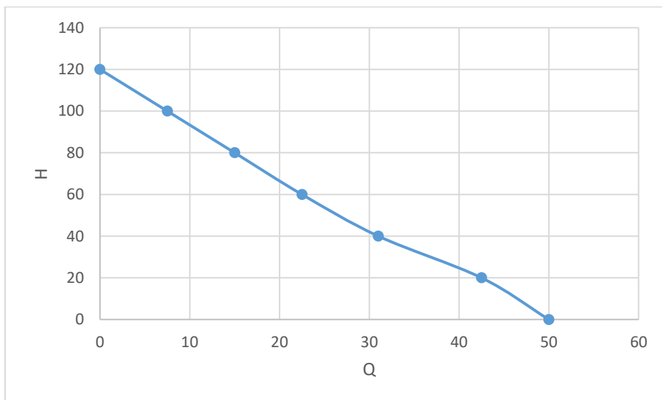
Caratteristica H (m col H 2 O) – Q (l/min) della pompa 4KSM 200
