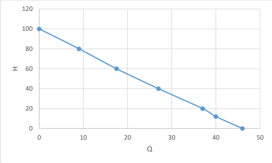
Características H (m col H2O) – Q (l/min) de la bomba 4KSM 150
