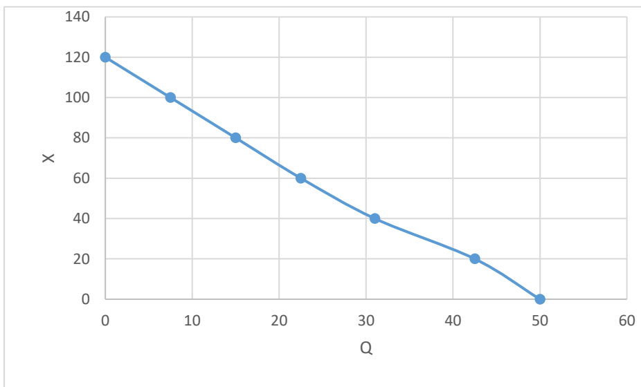
Χαρακτηριστικό H (m col H 2 O) – Q (l/min) στην αντλία 4KSM 200
