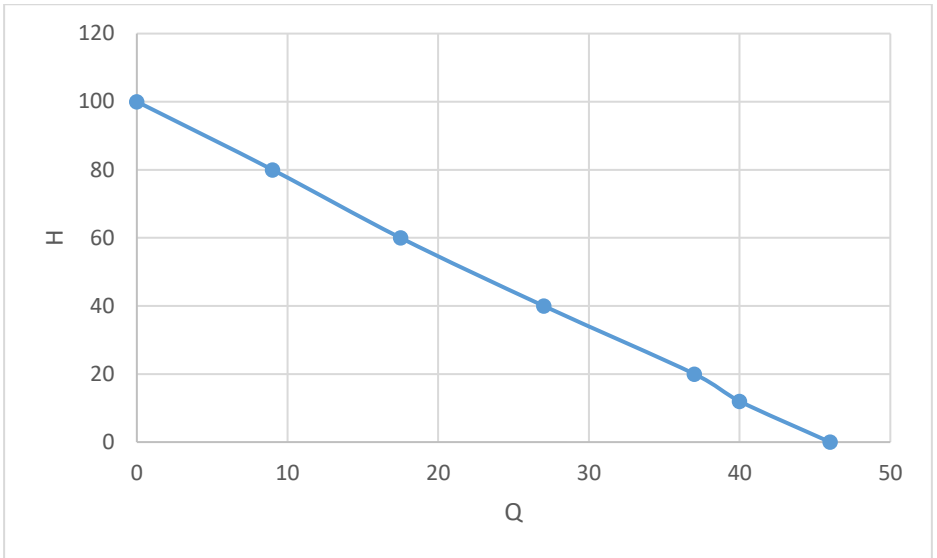
Caratteristica H (m col H 2 O) – Q (l/ min) a pompei 4KSM 150
