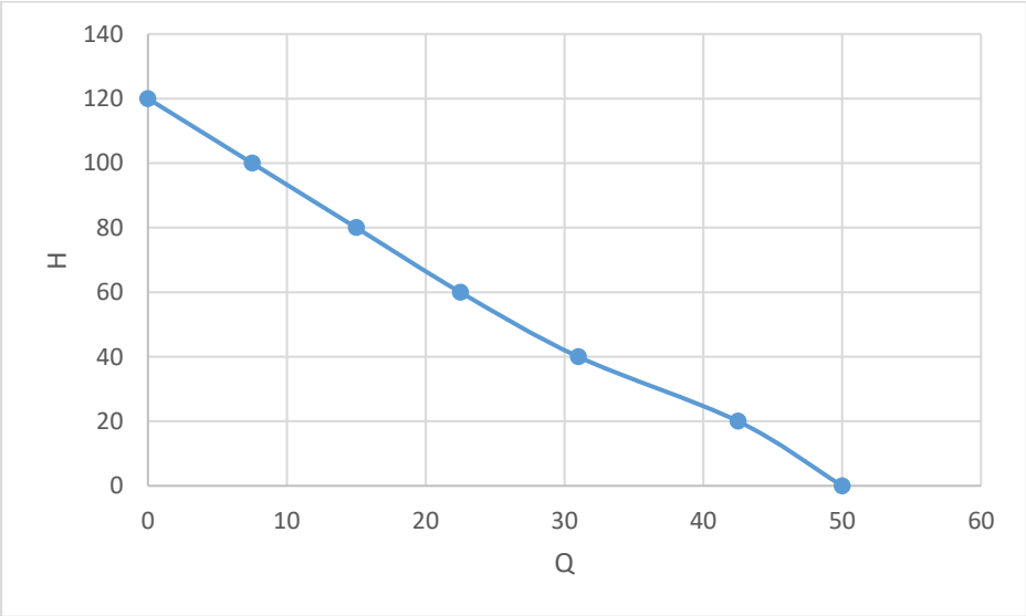
Característica H (m col H2O) – Q (l/min) da bomba 4KSM 200
