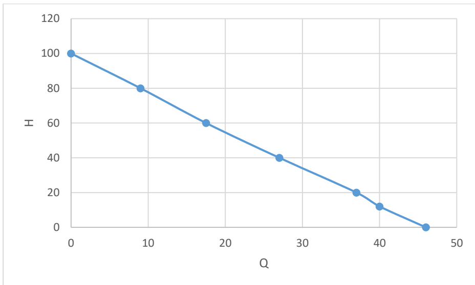
Caratteristica H (m col H 2 O) – Q (l/min) della pompa 4KSM 150
